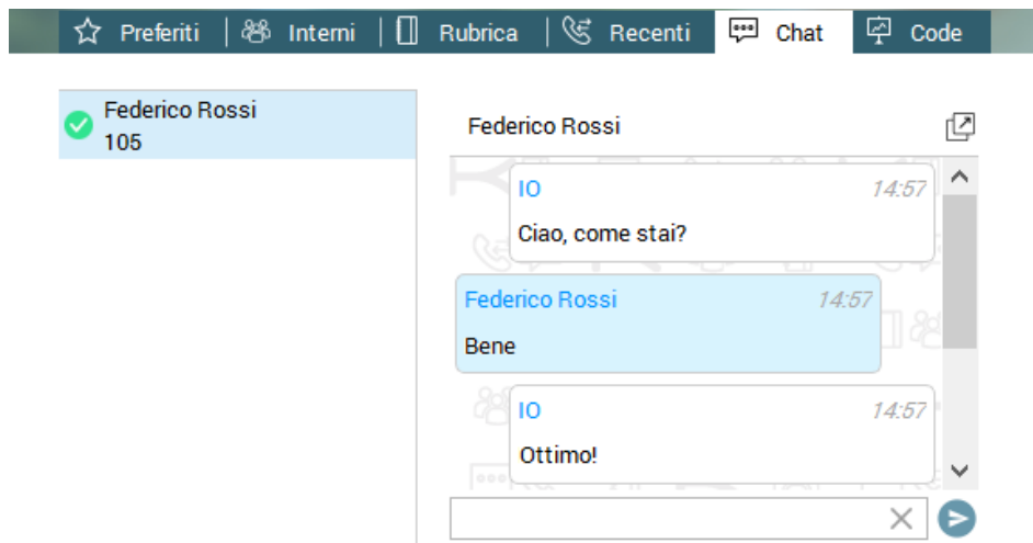
Figura 28 - Schermata Chat
